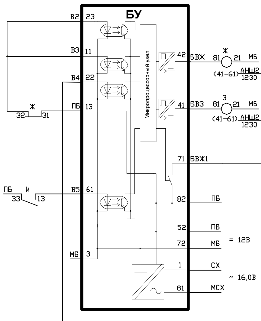
Рисунок 2 – Схема внешних подключений дешифратора ДА-3Ц на станции
