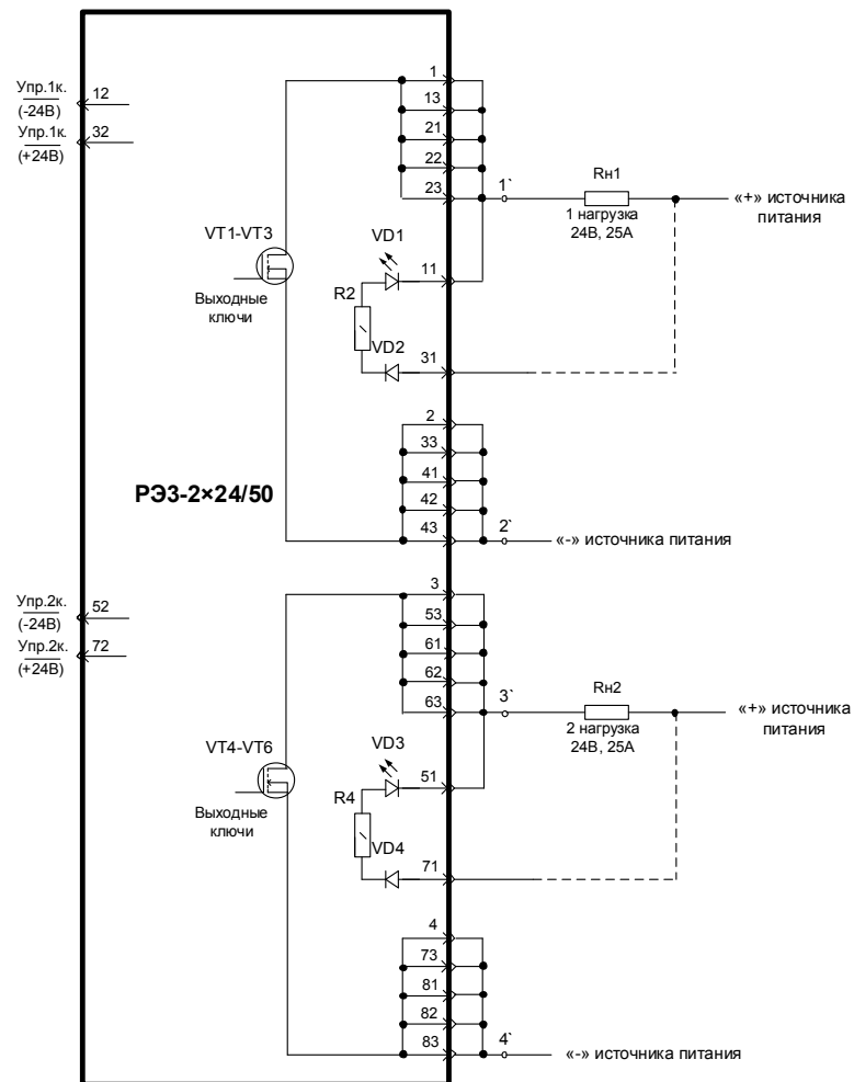
Рисунок 2 - Схема внешних подключений реле РЭЗ-2×24/50 при организации «минуса» к нагрузке
