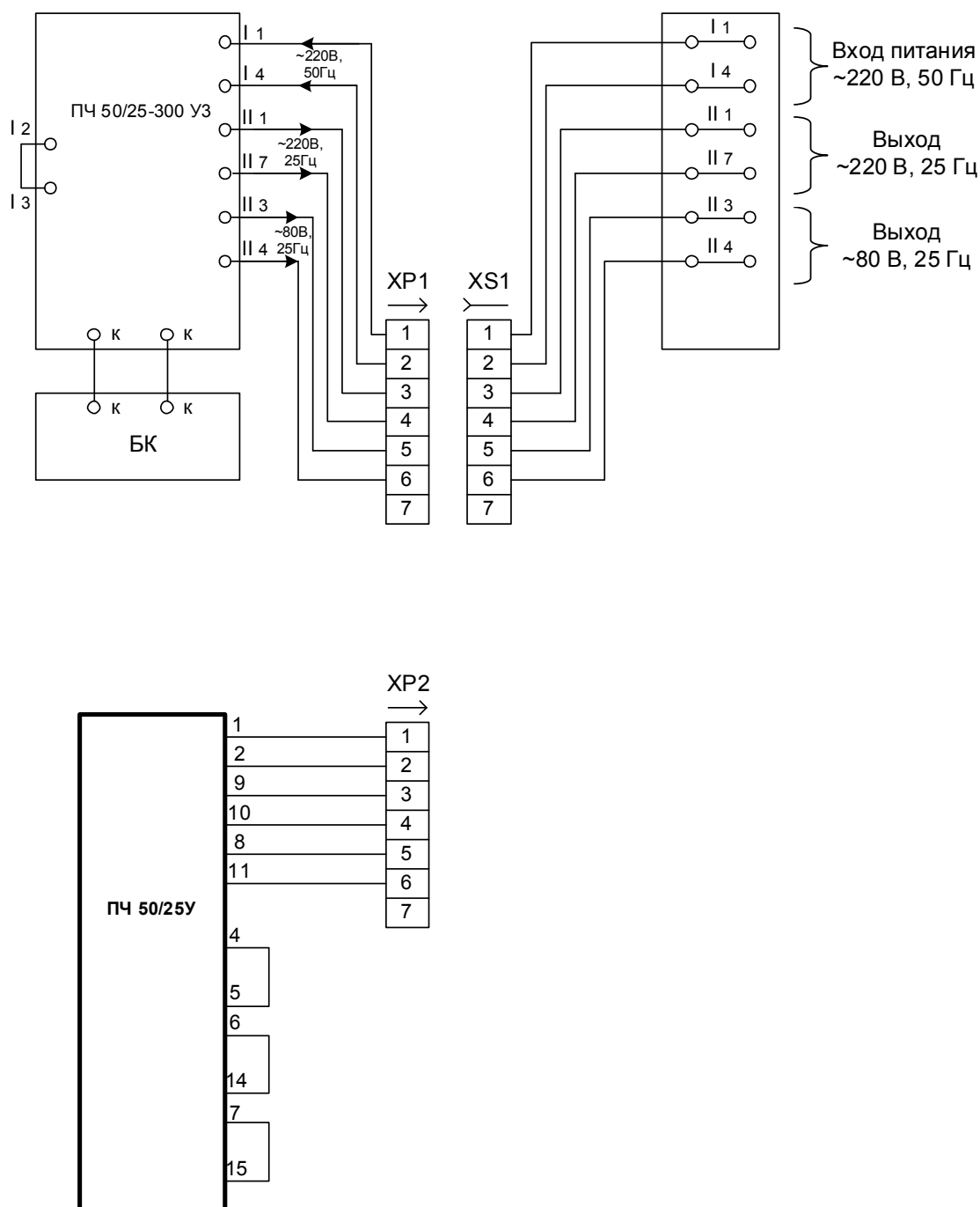
Рисунок 3 – Схема внешних подключений ПЧ 50/25У вместо ПЧ 50/25-300 УЗ при U_{\text{вых}} \sim 220 В частотой 25 Гц
