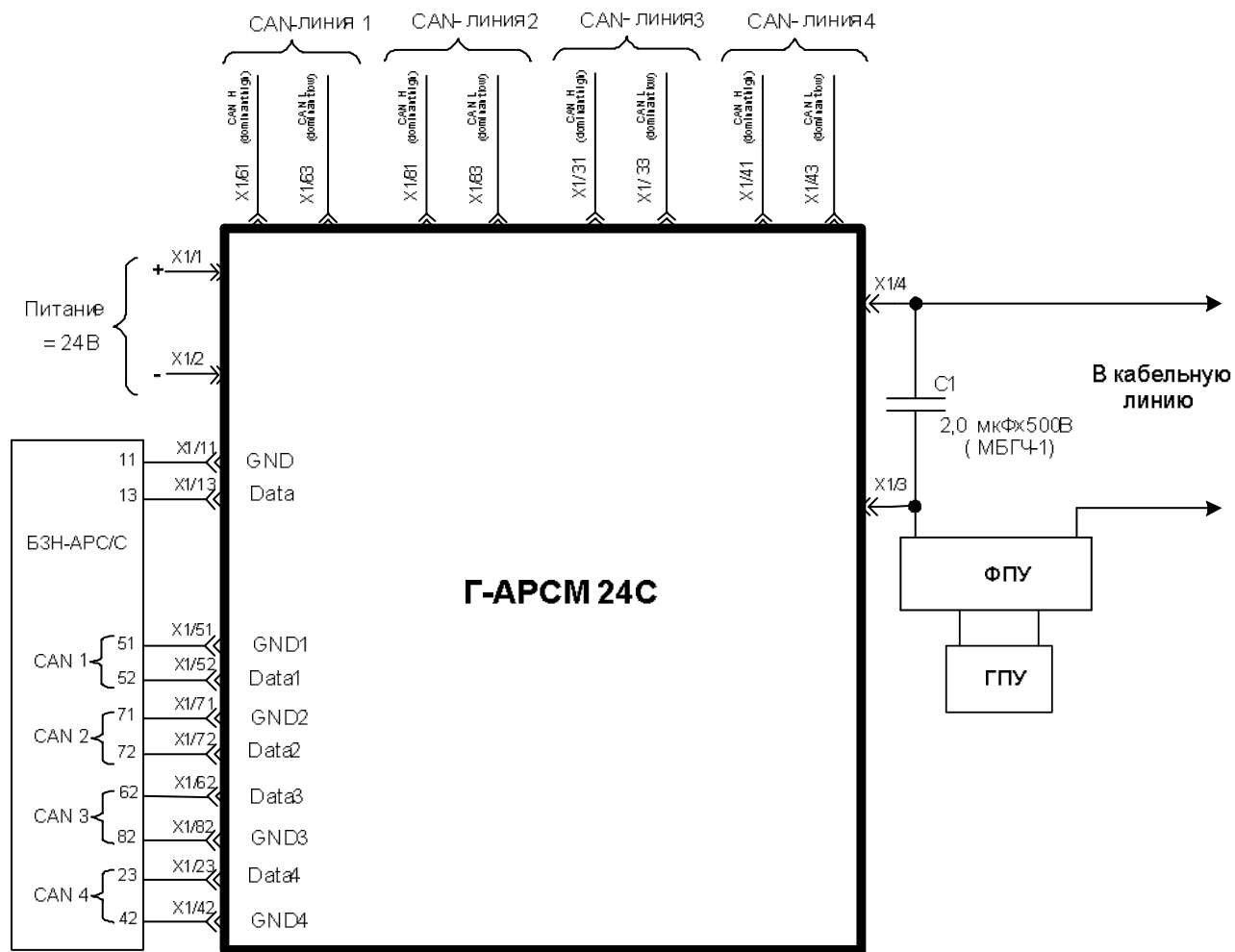
Рисунок 1 – Схема внешних подключений генератора Г-АРСМ 24С
