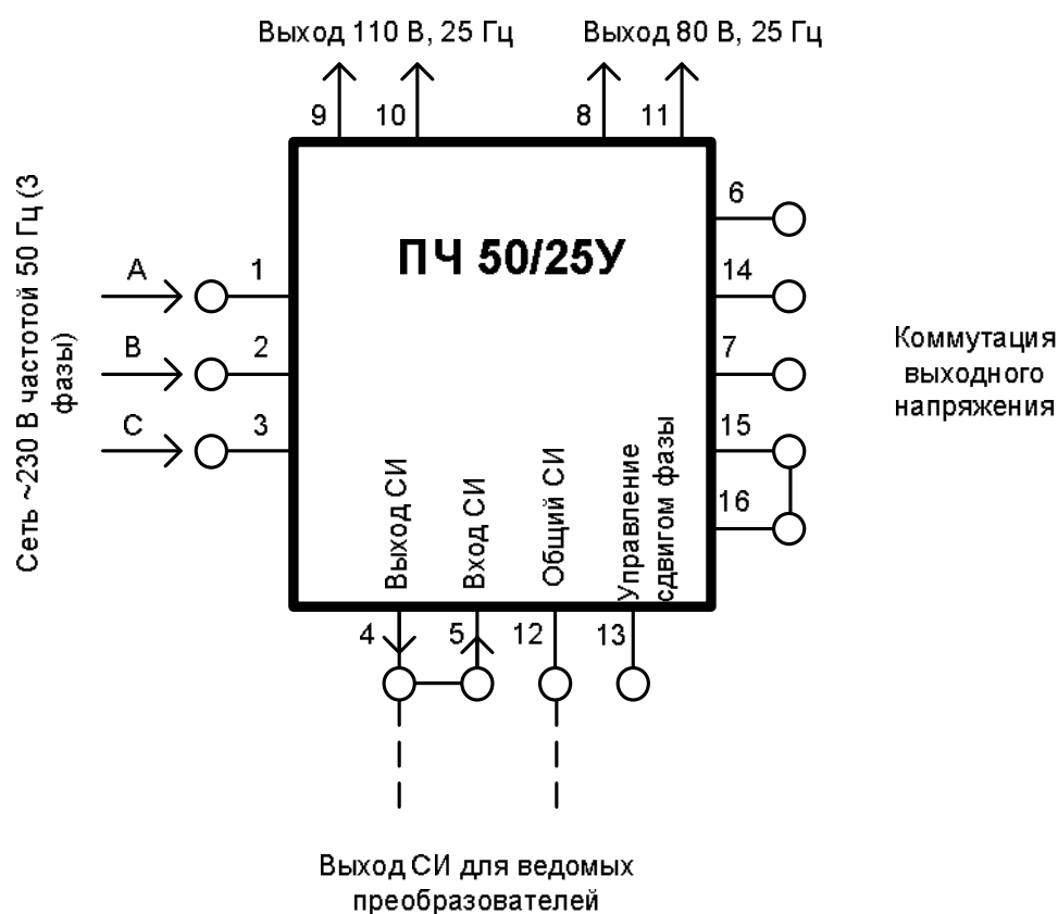
Рисунок 1 – Схема внешних подключений преобразователя ПЧ 50/25У при питании трехфазным напряжением, U_{\text{вых}} , 110 В частотой 25 Гц, с самосинхронизацией (в качестве ведущего), без фазового сдвига
