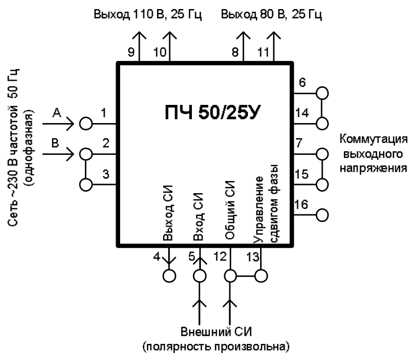
Рисунок 2 – Схема внешних подключений преобразователя ПЧ 50/25У при питании однофазным напряжением, U_{вых} , ~ 220 В частотой 25 Гц, с внешней синхронизацией (ведомый) и фазовым сдвигом
