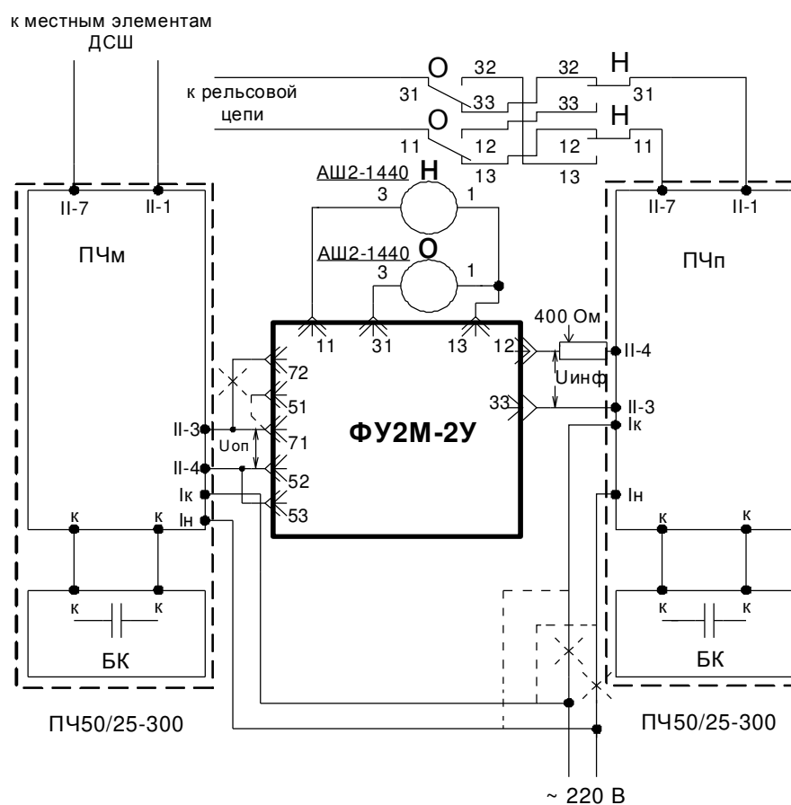
Рисунок 1 – Схема внешних подключений устройства ФУ2М-2У
