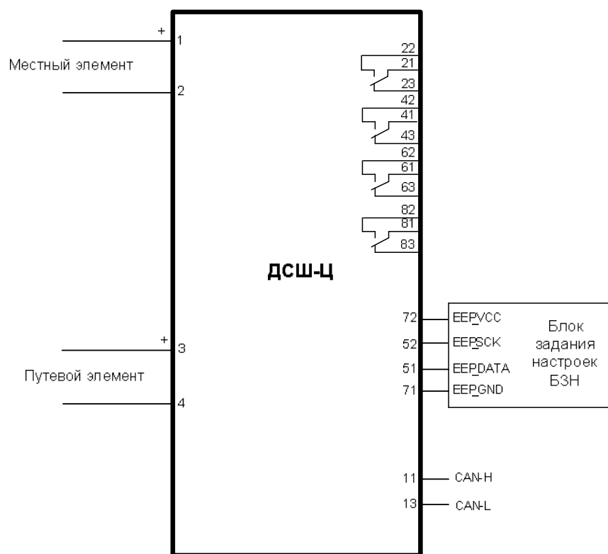
Рисунок 1 – Схема внешних подключений реле ДСШ-Ц
