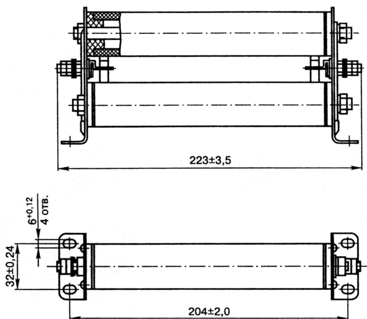
Рисунок 1 – Внешний вид и габаритные размеры резисторов РП
